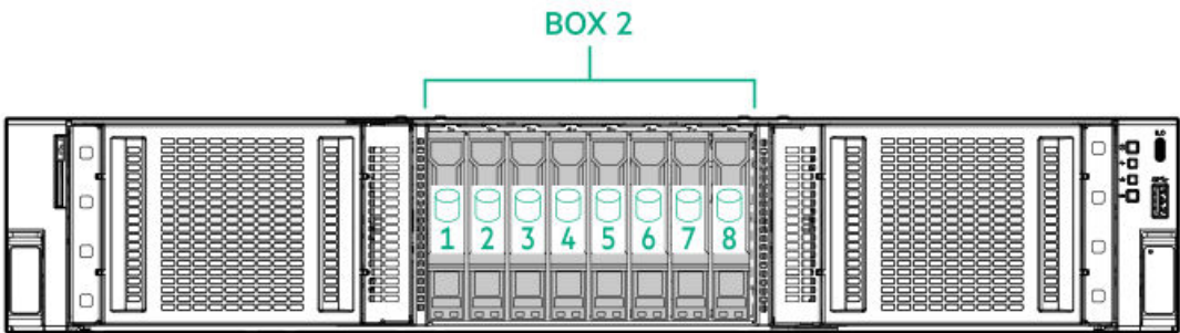
8SFF drive bay, GPU CTO server (P81949-B21)
